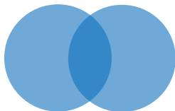
Venn Diagram
