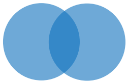
Venn Diagram
